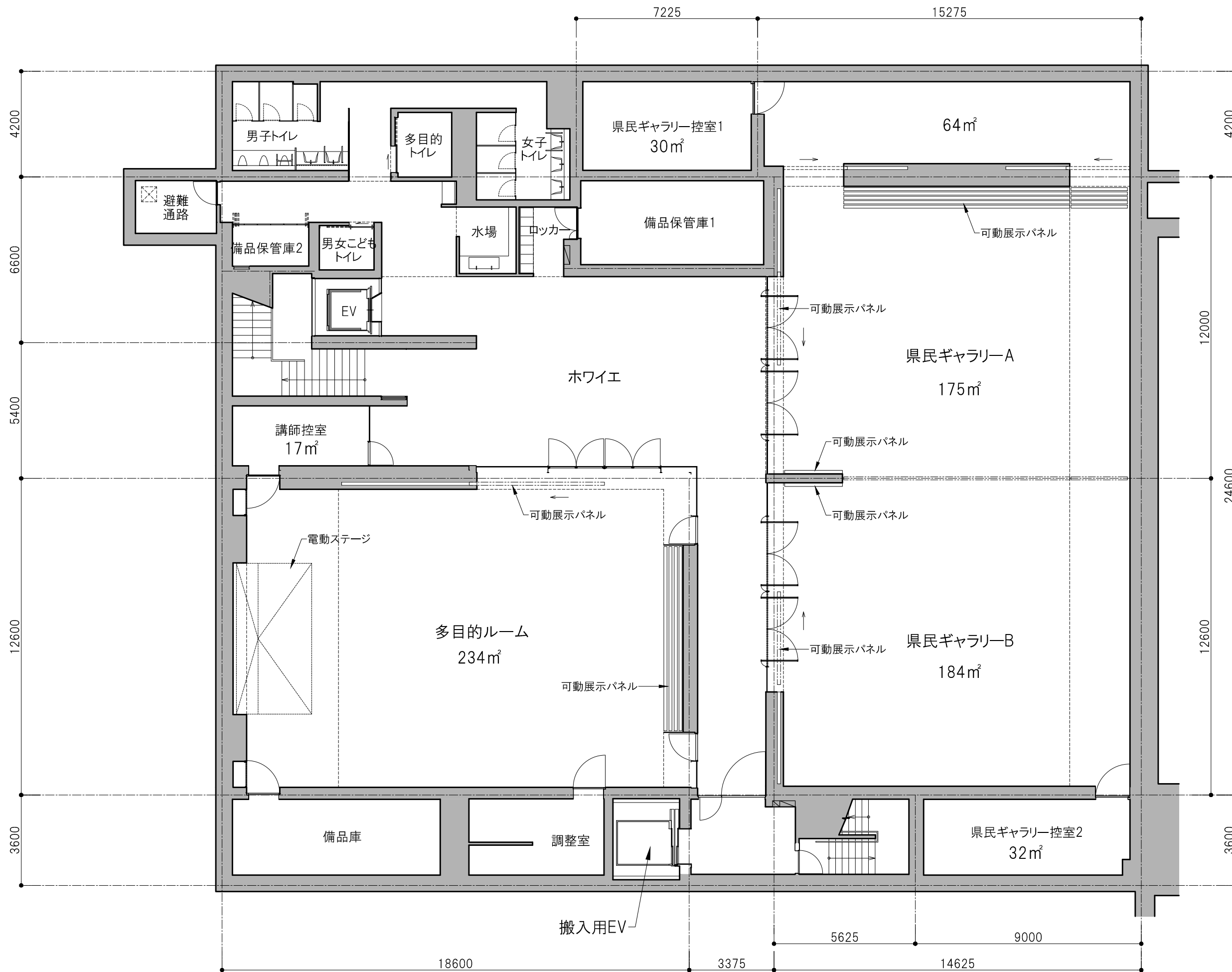
B1F 多目的ルーム・県民ギャラリー平面図 S=1:150(A3)
